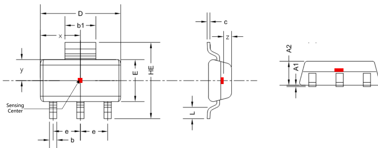
图.16 SOT-89B 封装图
