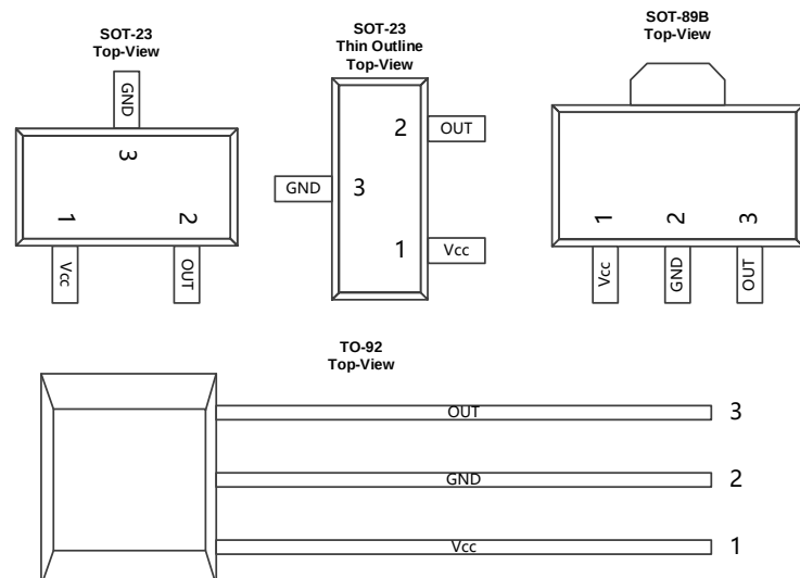
图.1 引脚配置和功能
